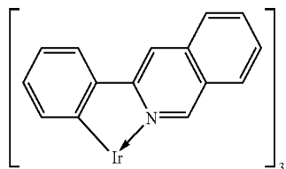
Ir(p-3iq) 3
